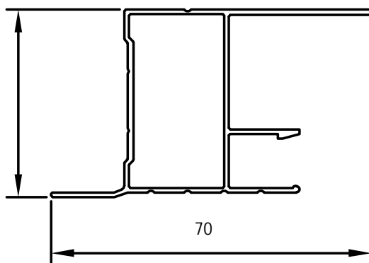
Vinduesramme profil
