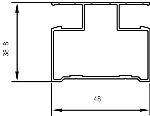
Dørramme profil
