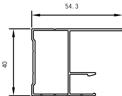
Vinduesramme profil
