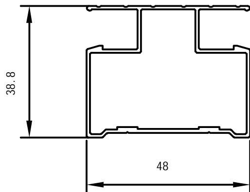
Dørramme profil
