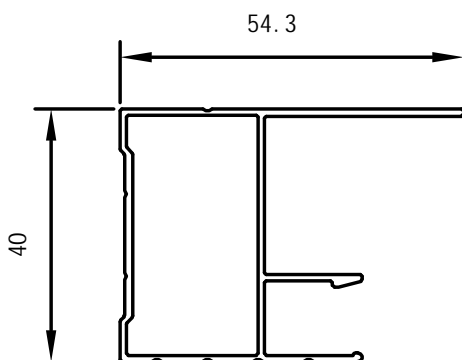
Vinduesramme profil
