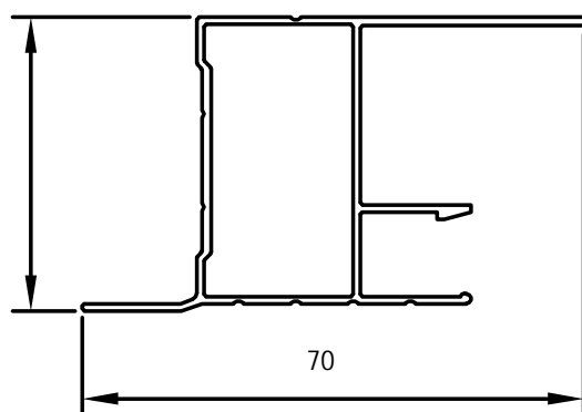
Vinduesramme profil
