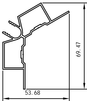
Tag profil
