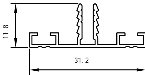
Tryk dæksel dobbelt
