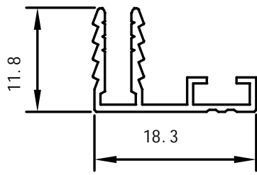
Tryk dæksel single
