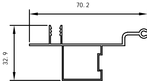
Vindues profil
