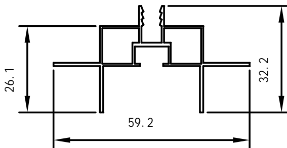
Stolpe profil ved dør
