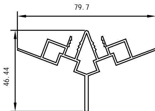
Skotrende profil
