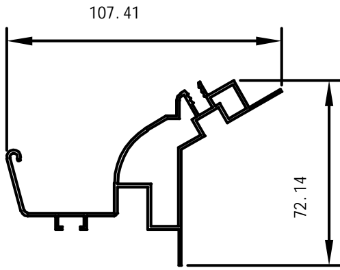
Tagrende profil
