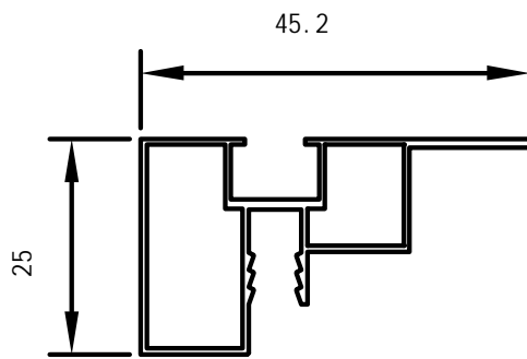
Sokkel profil
