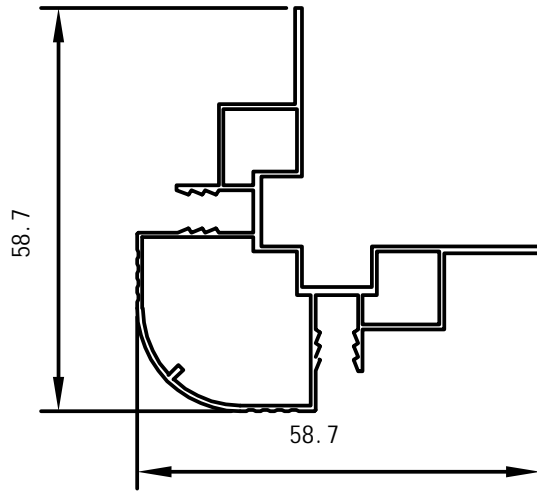
Hjørnestolpe profil
