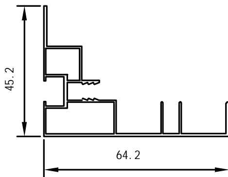
Sokkel ved skydedør
