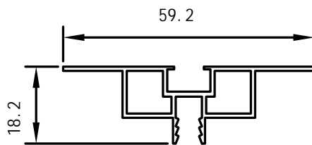
Mellemstolpe profil
