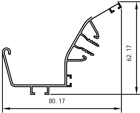
Tagrende profil
