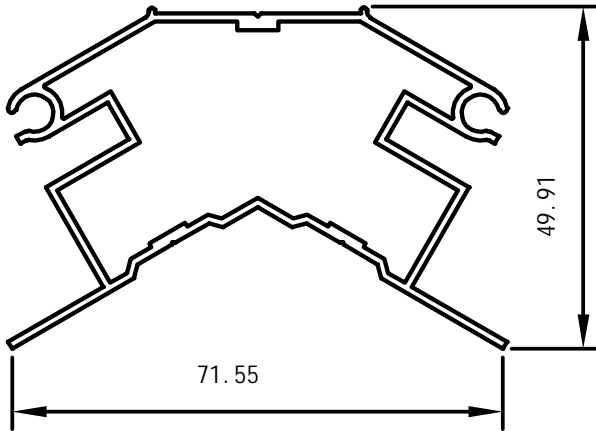
Tagryg profil
